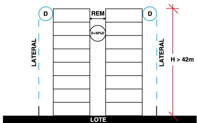
CORTE ESQUEMÁTICO
